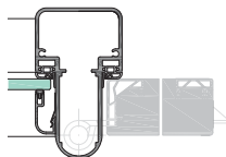
KFI Pfostenprofil
