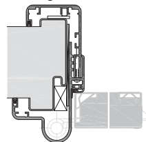
RENOFI Renovierungszarge
